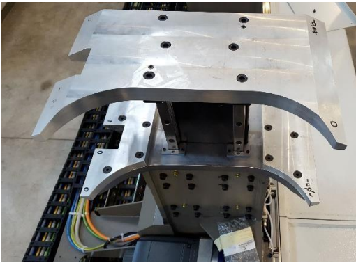
MAGAZIE DE SCULE TIP DEPLASABILA CU 128 POZITII – INTERAXE 105 MM
